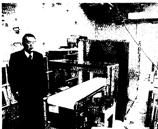
アドバンスフードテックが開発した磁性金属異物検出装置
